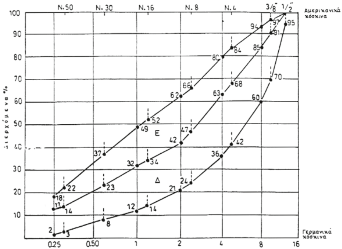
Διάγραμμα III : Όρια κοκκομετρικής διαβαθμίσεως μίγματος αδρανών μέγιστου κόκκου □ 16 ή 1 1/2".
